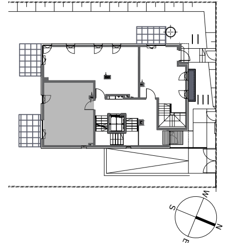
SCHEMAT KONDYGNACJI
